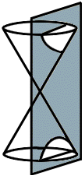
Hyperbola
