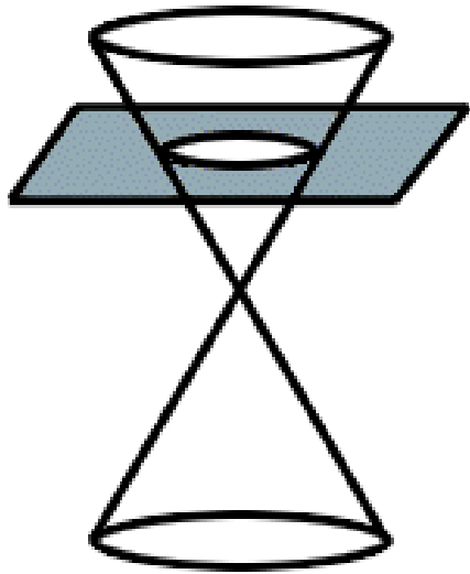
Circle
