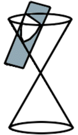
Parabola
